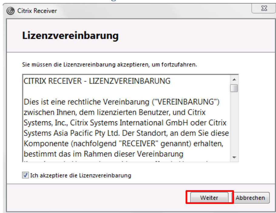
Abbildung 1 - Lizenzvereinbarung bestätigen
