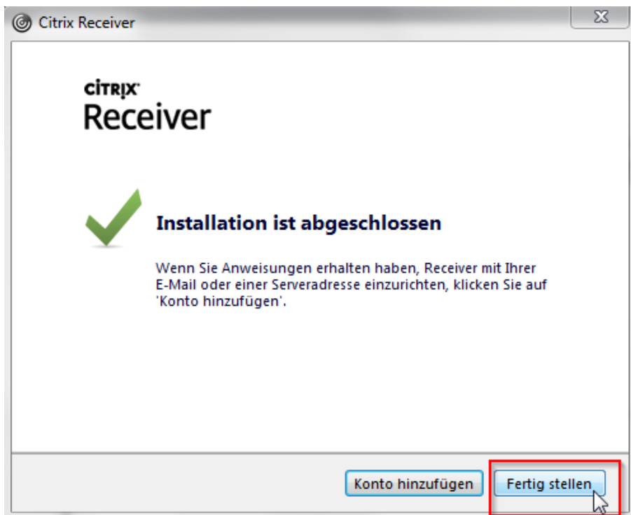
Abbildung 3 - Fertig stellen
